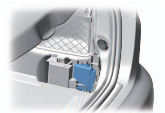
Einbauort des Steuergeräts für Parklenkassistent J791 im Audi A3 Sportback.
