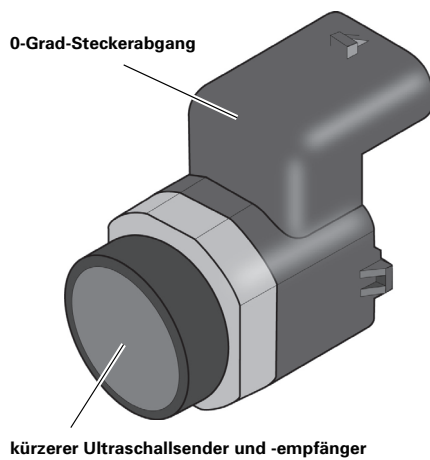
Ultraschallsensor für akustische Einparkhilfe
