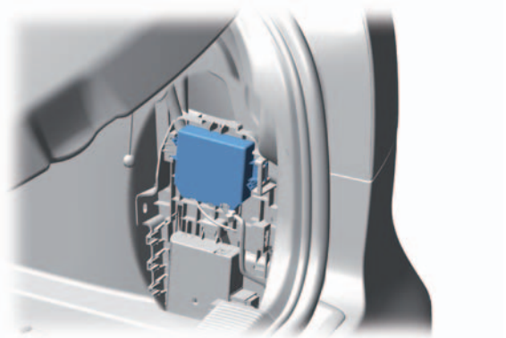
Einbauort des Steuergeräts für Parklenkassistent J791 im Audi A3.
